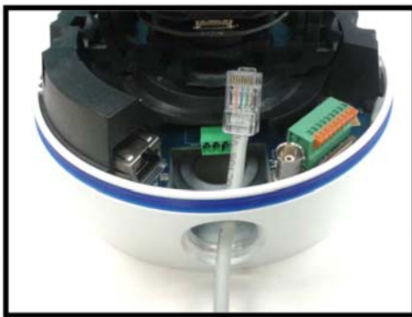
Side Conduit Entry
