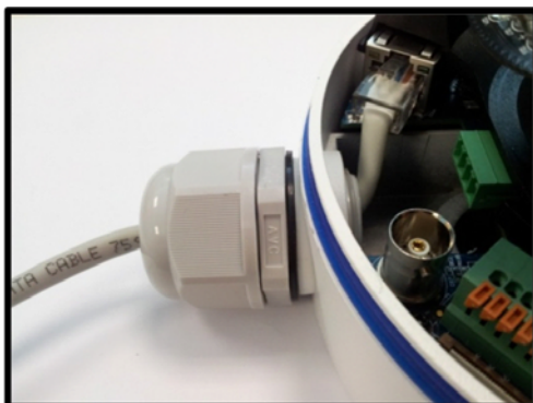
Side Conduit Entry
